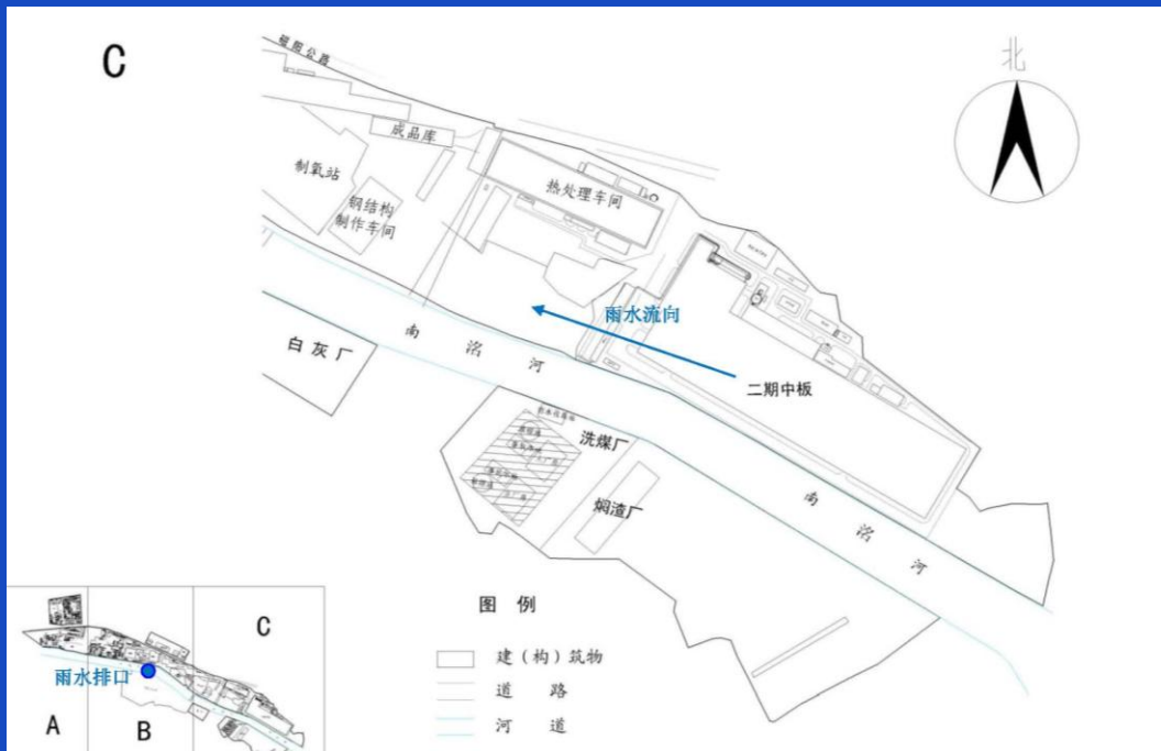
全厂平面布置图
